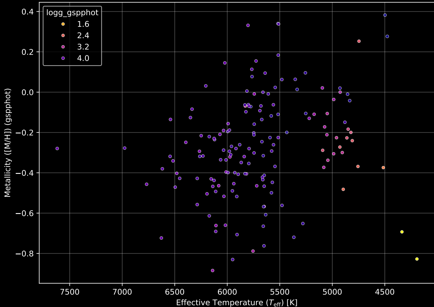
GALAH DR4 Field: [7211] Stellar Population Parameters (n= 155)
